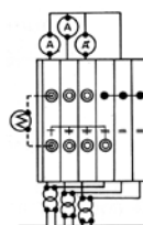
PROVA T.A. TRIFASE CONCATENATO
